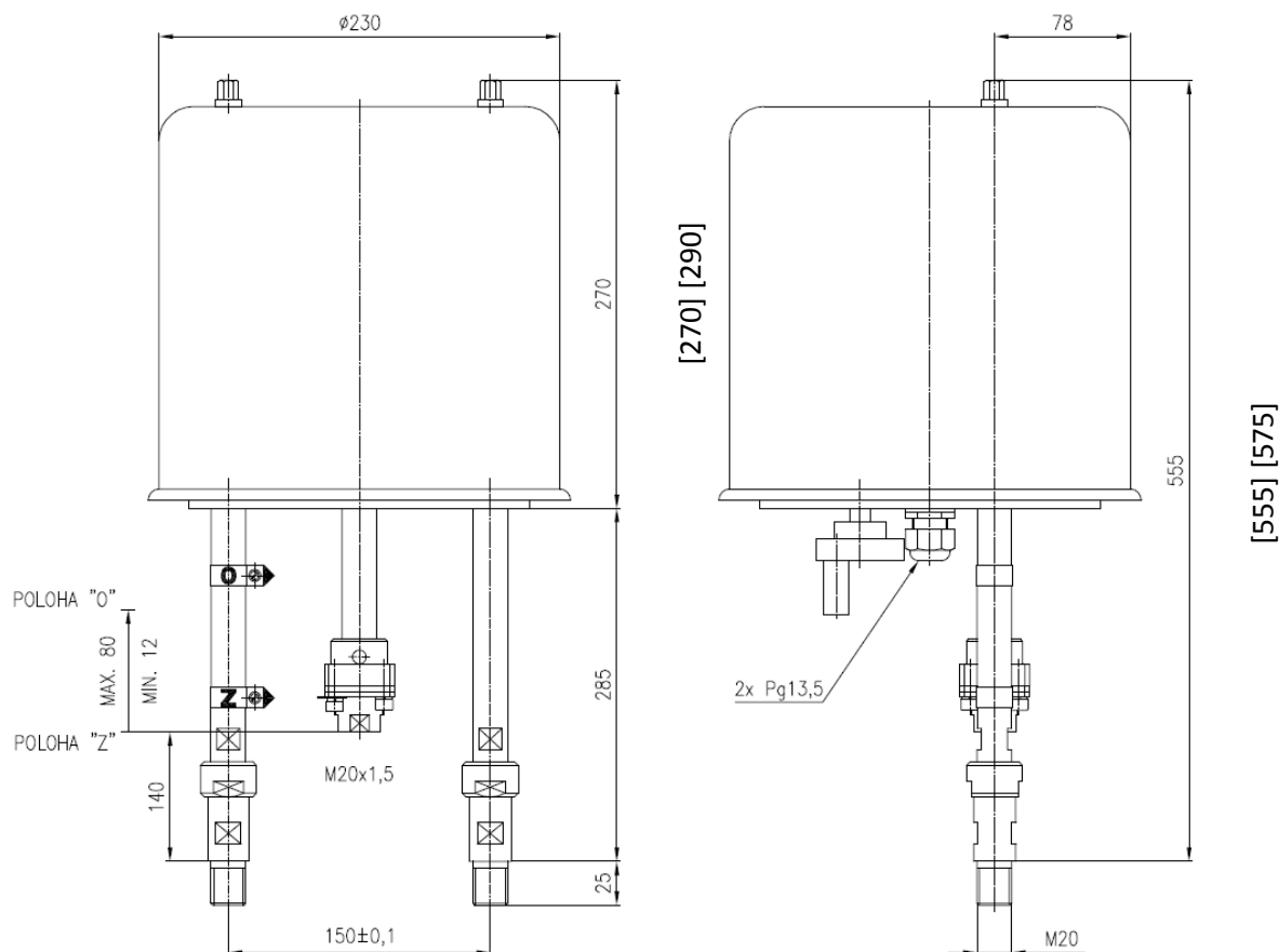
8.1. Rozměrový nákres – připojení PTN7.XX.XX.XX.30
