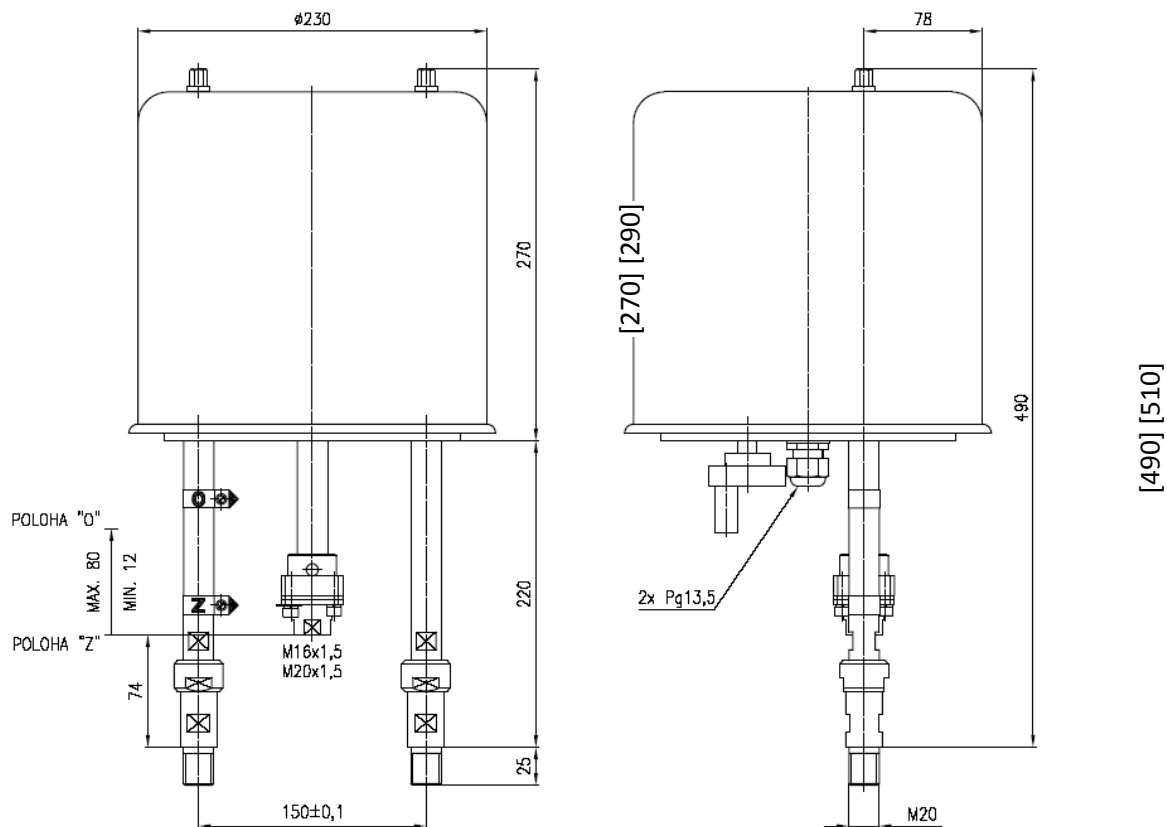
8.1. Rozměrový nákres – připojení PTN7.XX.XX.XX.10 PTN7.XX.XX.XX.20
