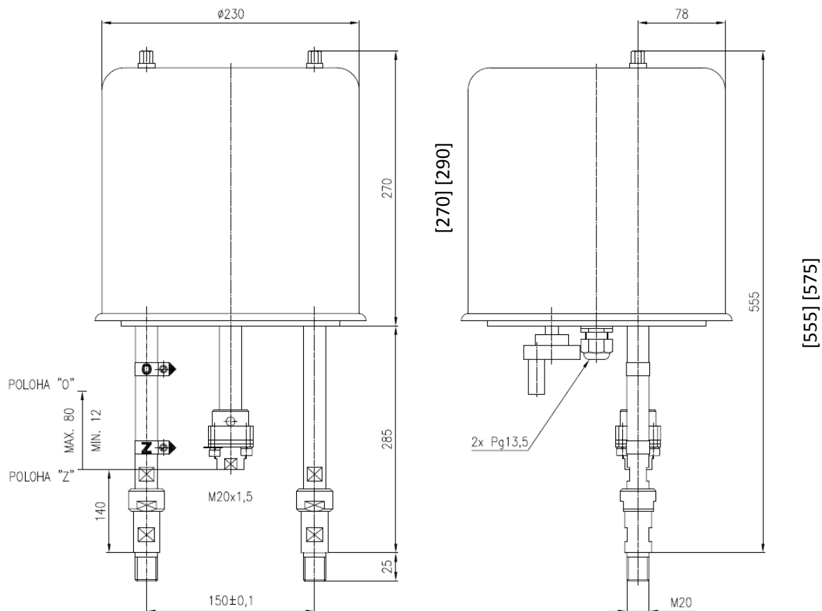
7.1. Rozměrový nákres – připojení PTN7.XX.XX.XX.30
