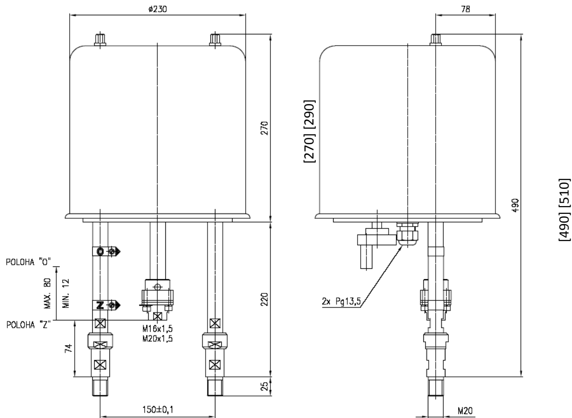
7.1. Rozměrový nákres – připojení PTN7.XX.XX.XX.10 PTN7.XX.XX.XX.20
